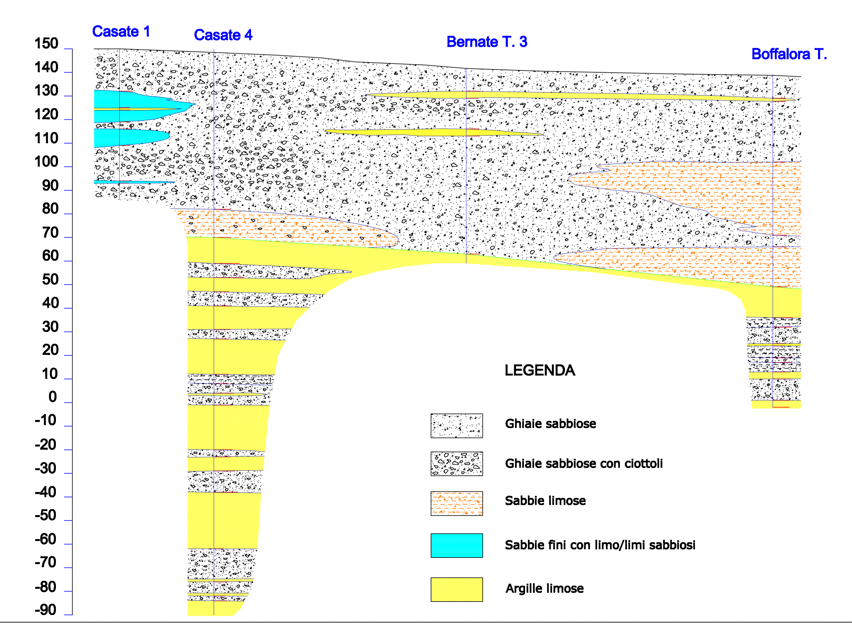
SEZIONE LITOSTRATIGRAFICA - Scala 1:10.000/1.000
